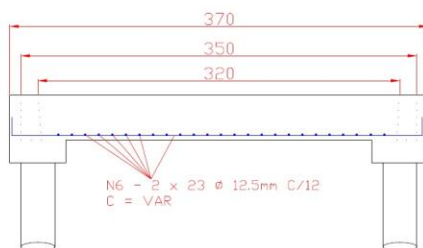
Corte "AA" - Detalhe armadura da laje Escala 1:25
