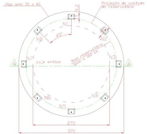
Forma do bloco/ localização do Nichos Escala 1:25
