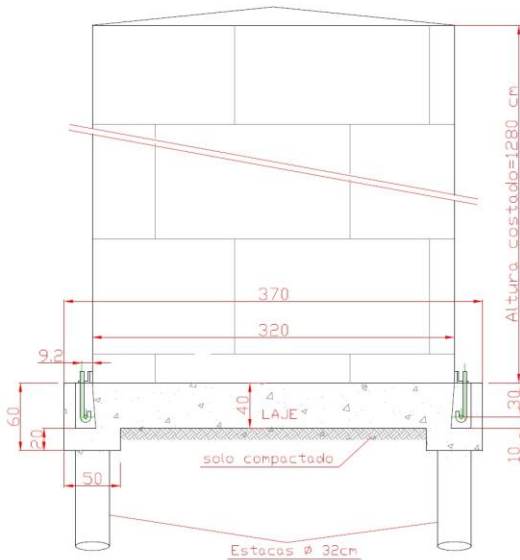
Corte "AA" Escala 1:25
