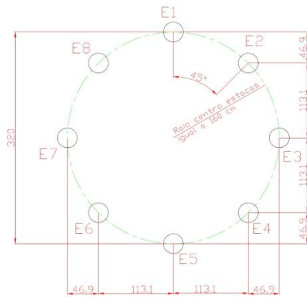
locação das estacas Escala 1:25
