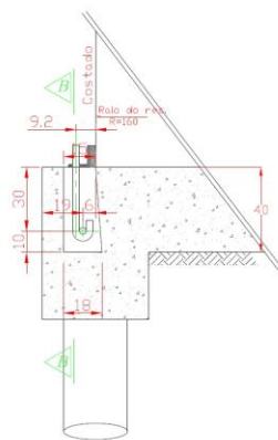
Corte "AA" Sem escala
