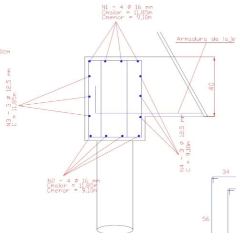
Detalhe engaste das Estacas 1/2 escala
