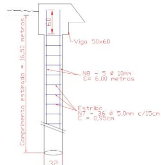
Detalhe engaste das Estacas 1/2 escala
