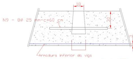
Corte "BB" Sem escala
