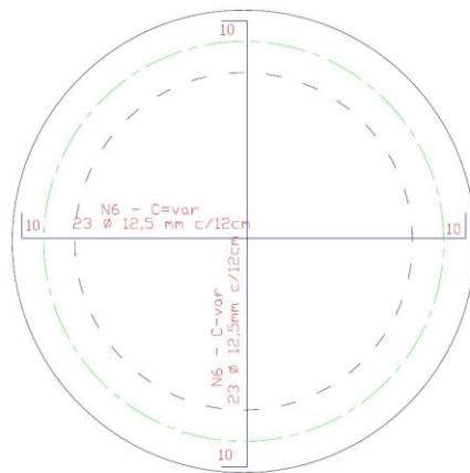
Planta - Armadura da laje Escala 1:25
