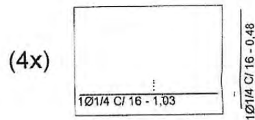
ARMADURA LAJE SUPERIOR
