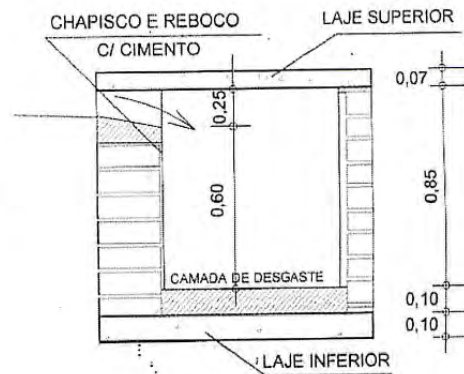
CORTE AA
