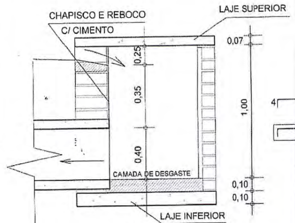
CORTE BB
