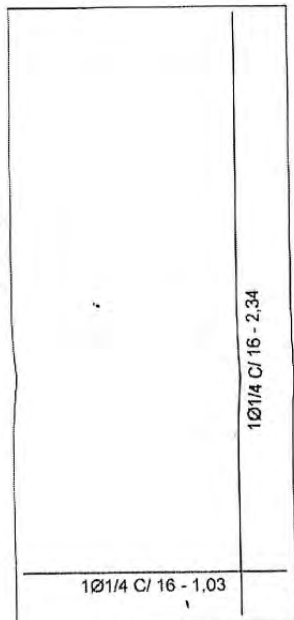
ARM. LAJE INFERIOR
