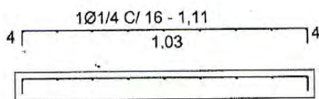
ARM. LAJE INFERIOR
